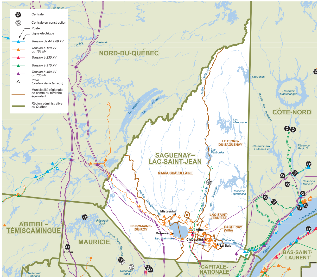
Carte du réseau électrique d'Hydro-Québec en 2005 Source des limites administratives : Ministère des ressources naturelles – SDA, janvier 2006
