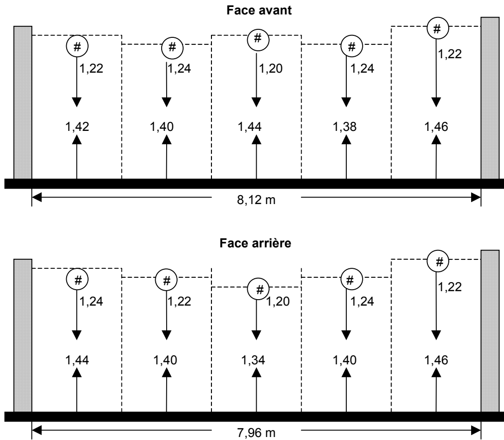
Figure 71 Exemple de calcul du volume apparent
