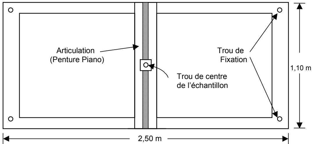
Figure 73 Gabarit pour un Échantillon rectangulaire
