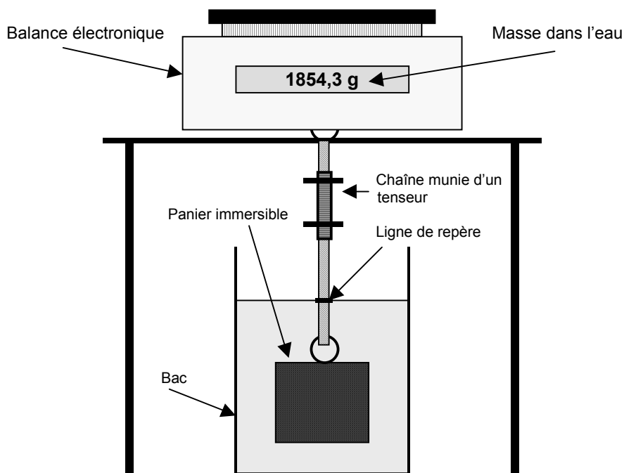
Figure 86 Outillage requis pour mesurer les copeaux
