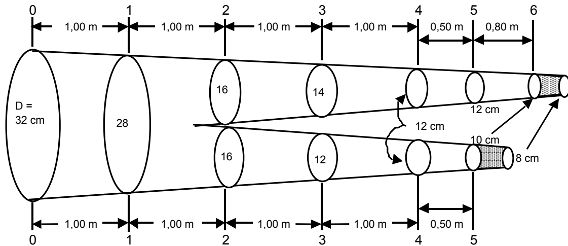
Figure 77 Tige fourchue avec branches inégales
