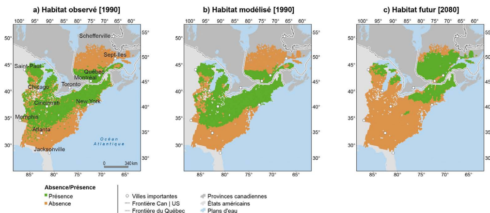
Figure 2. Illustration des résultats de la modélisation pour l'érable à sucre dans l'est de l'Amérique du Nord. Les zones en vert illustrent la présence probable de conditions favorables à l'espèce pour a) l'habitat observé, b) l'habitat modélisé et c) l'habitat futur. Les probabilités ont été calculées pour 6 418 pixels de 400 km 2 .
