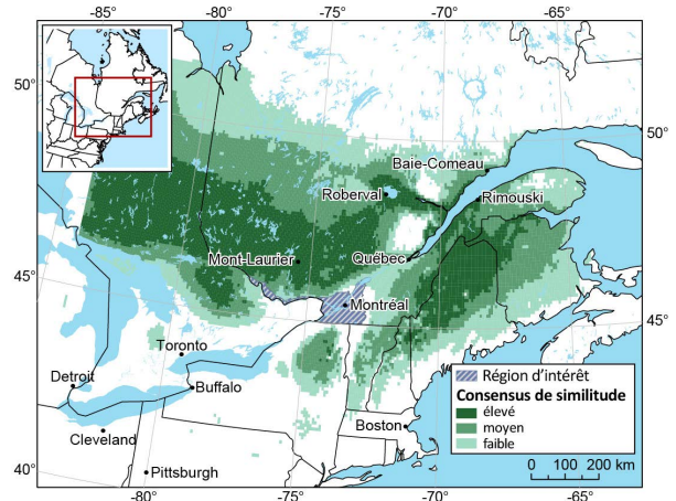
Figure 1. Analogues climatiques de la région de Montréal à la fin du 21 e siècle (2071-2100), construits à partir des projections de la température annuelle moyenne et des précipitations totales annuelles de 139 scénarios climatiques (1971-2000). Adapté de Logan (2014).
