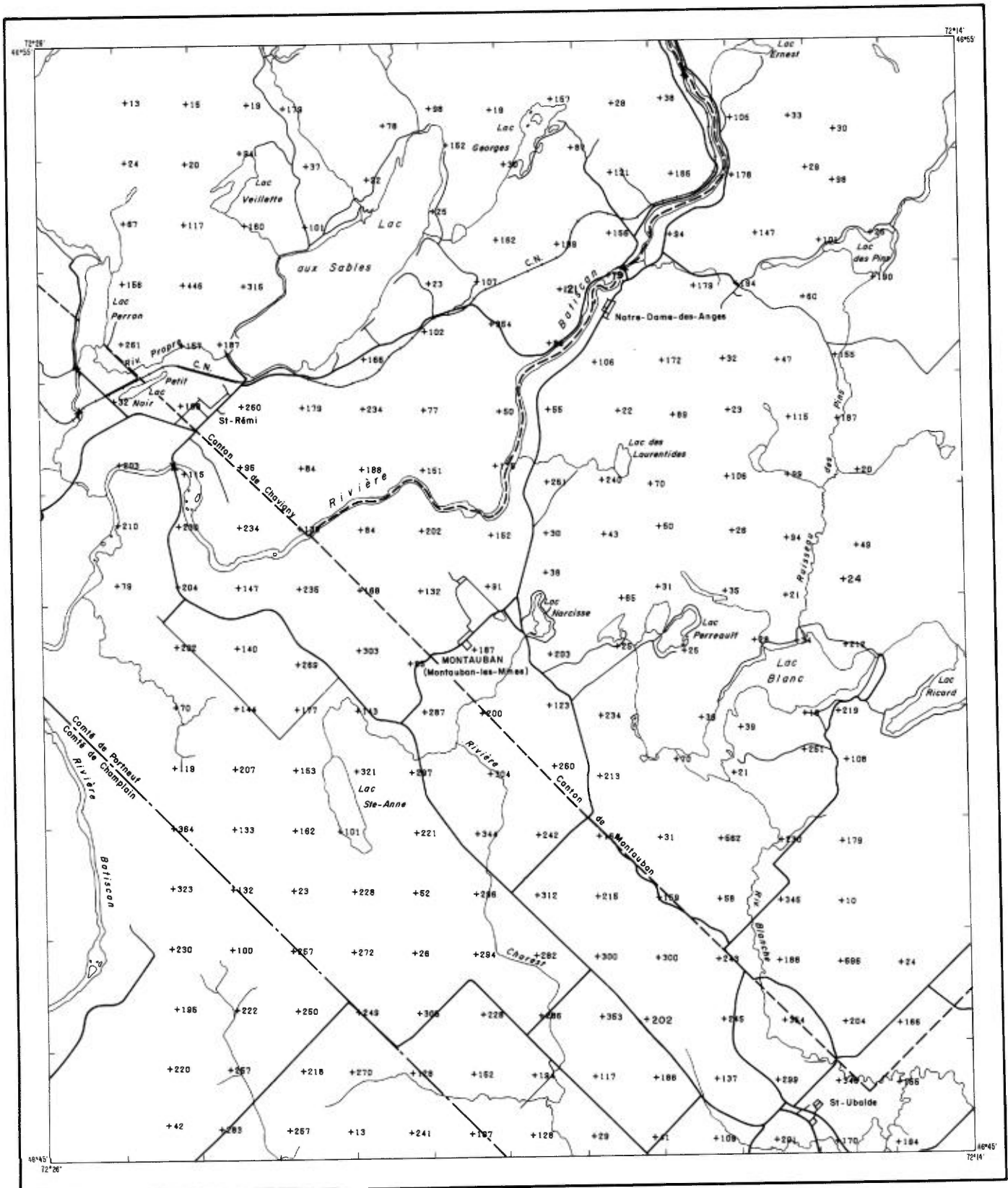
FIGURE 19 - Carte géochimique - Fe (pct x 100)
