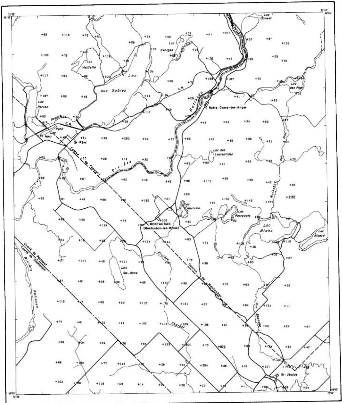
FIGURE 6 - Carte géochimique - Zn (ppm)
