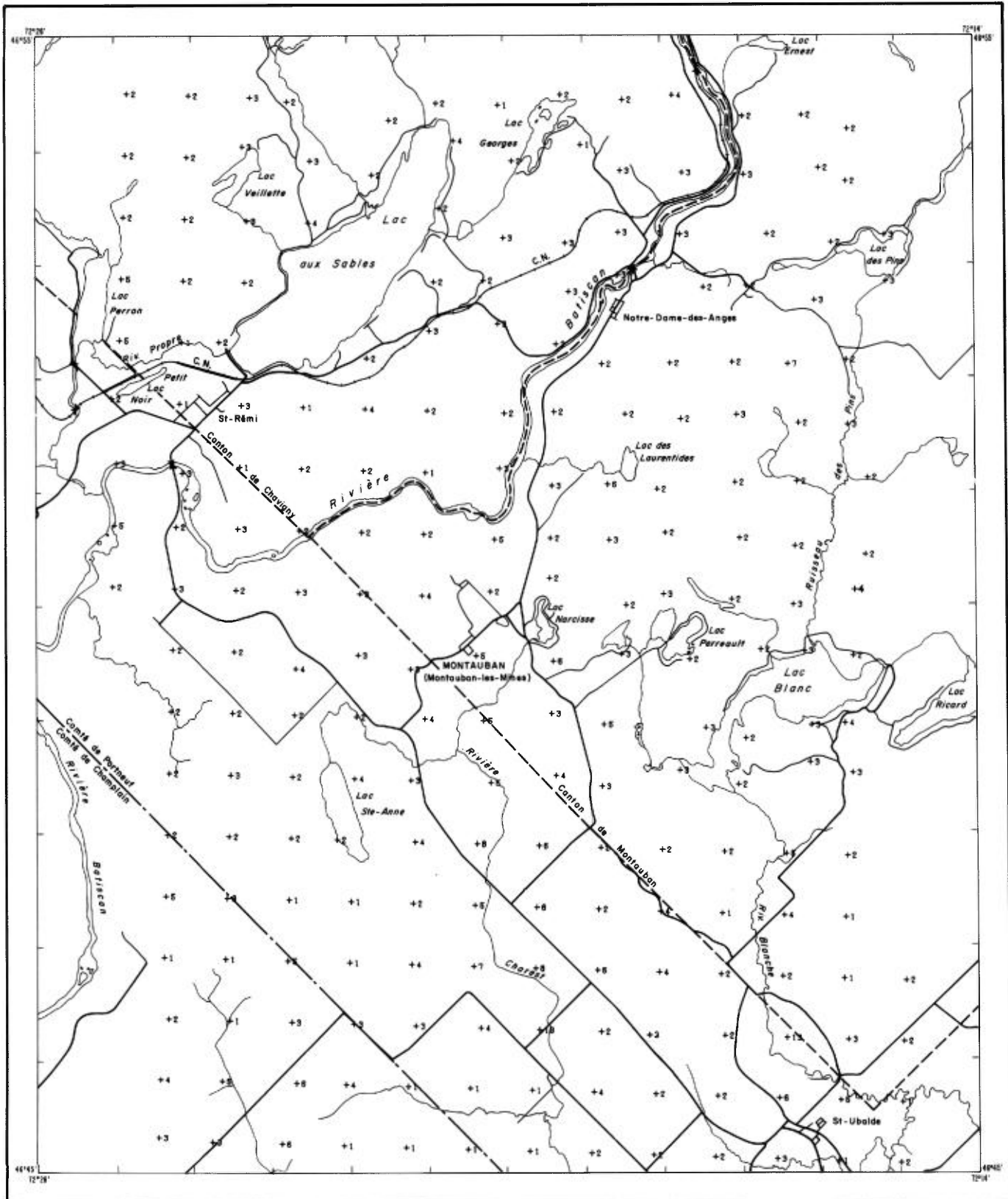
FIGURE 12 - Carte géochimique - Na (pct x 100)
