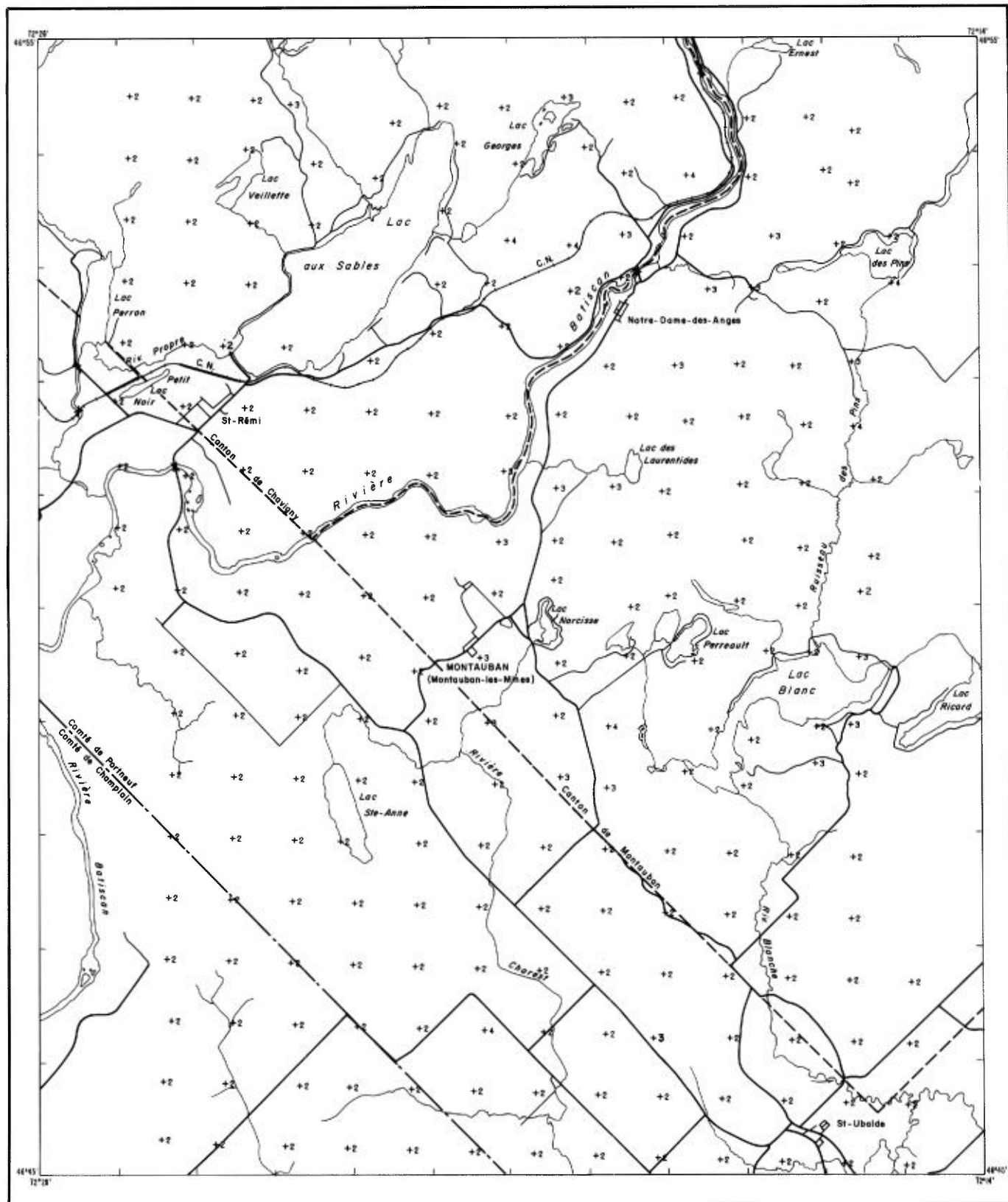
FIGURE 33 - Carte géochimique - Be (ppm)
