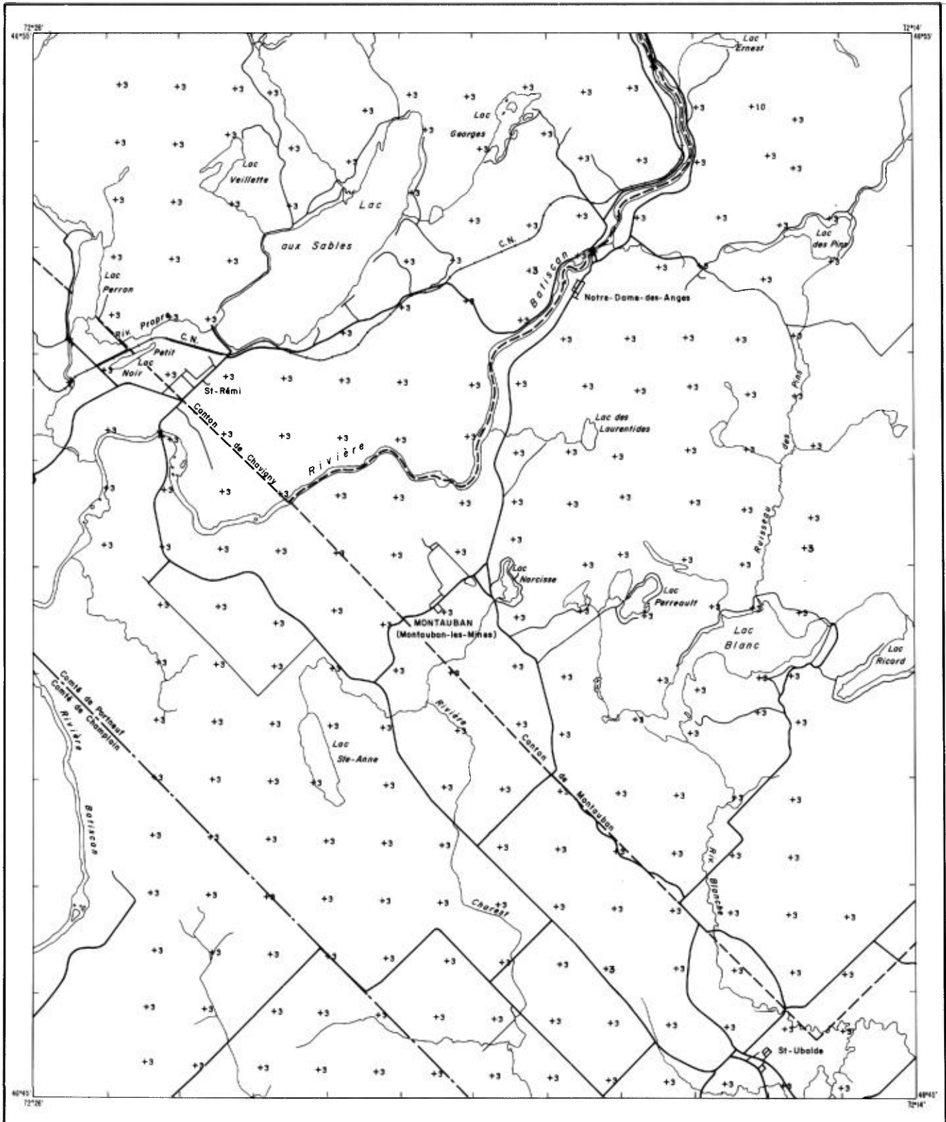
FIGURE 29 - Carte géochimique - Mo (ppm)
