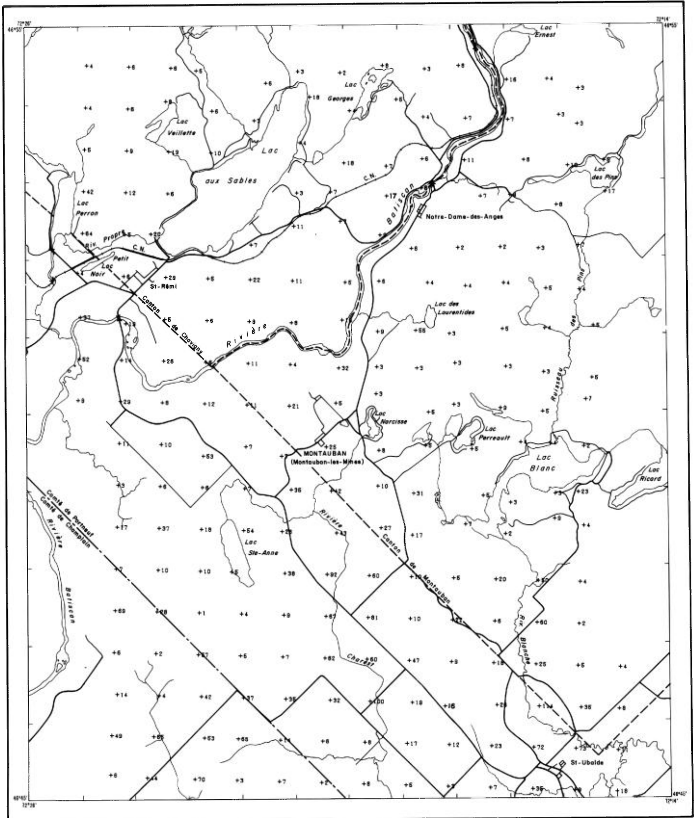
FIGURE 32 - Carte géochimique - Mg (pct x 100)
