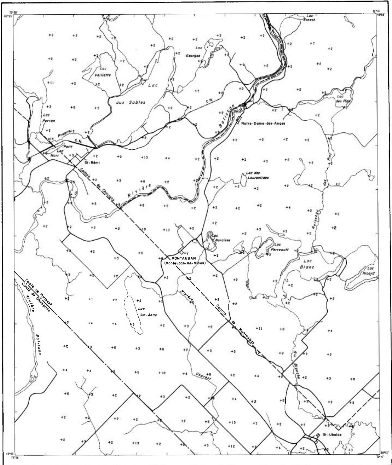
FIGURE 10 - Carte géochimique - Cd (ppm x 10)
