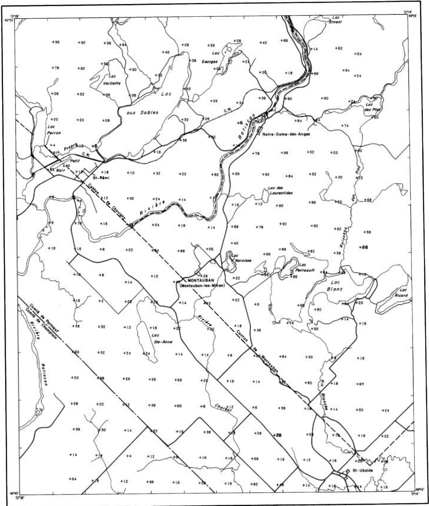
FIGURE 34 - Carte géochimique - PF (pct)
