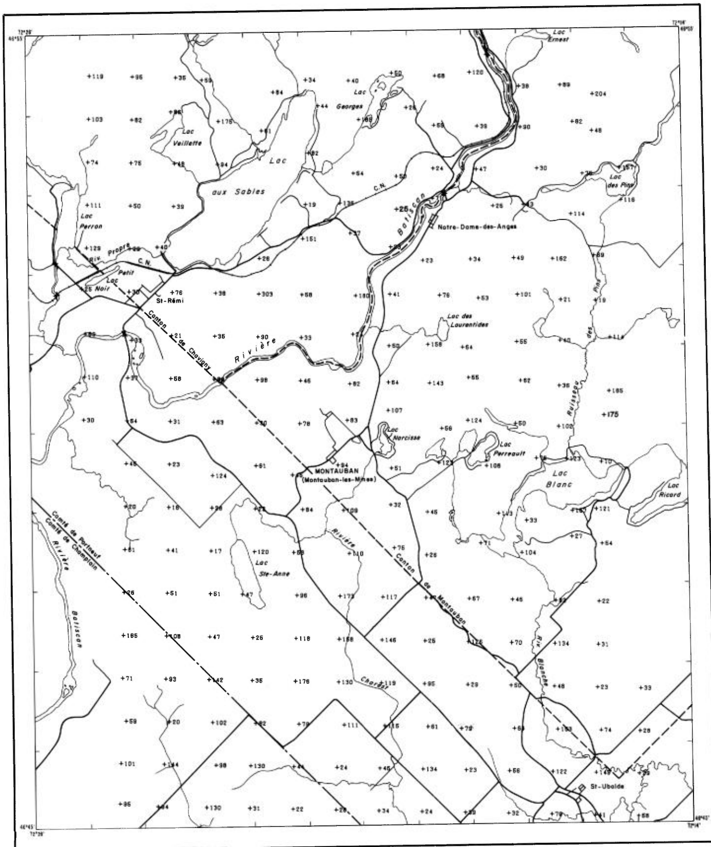
FIGURE 27 - Carte géochimique - Ba (ppm)
